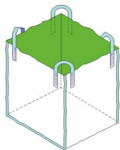
asole incrociate agli angoli
